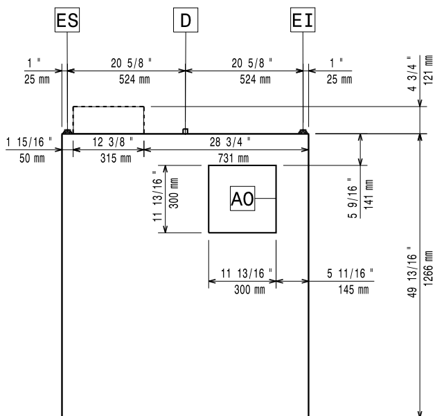
Planta
